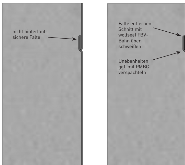
Instandsetzung einer Falte nach dem Ausschalen
