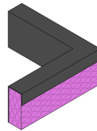
thepro DDS Außenecke Außenschenkel: 1,20 lfm + Dämmstoffstärke Dämmstärken: 80 - 200 mm Höhe: 20, 25, 30, 35, 40, 60 cm
